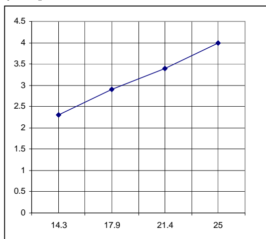
Фигура 2. Зависимост на параметрите за настройка (времето за подаване на гориво – T4 и отношението T4/T6 ) от топлинната мощност на котела;
