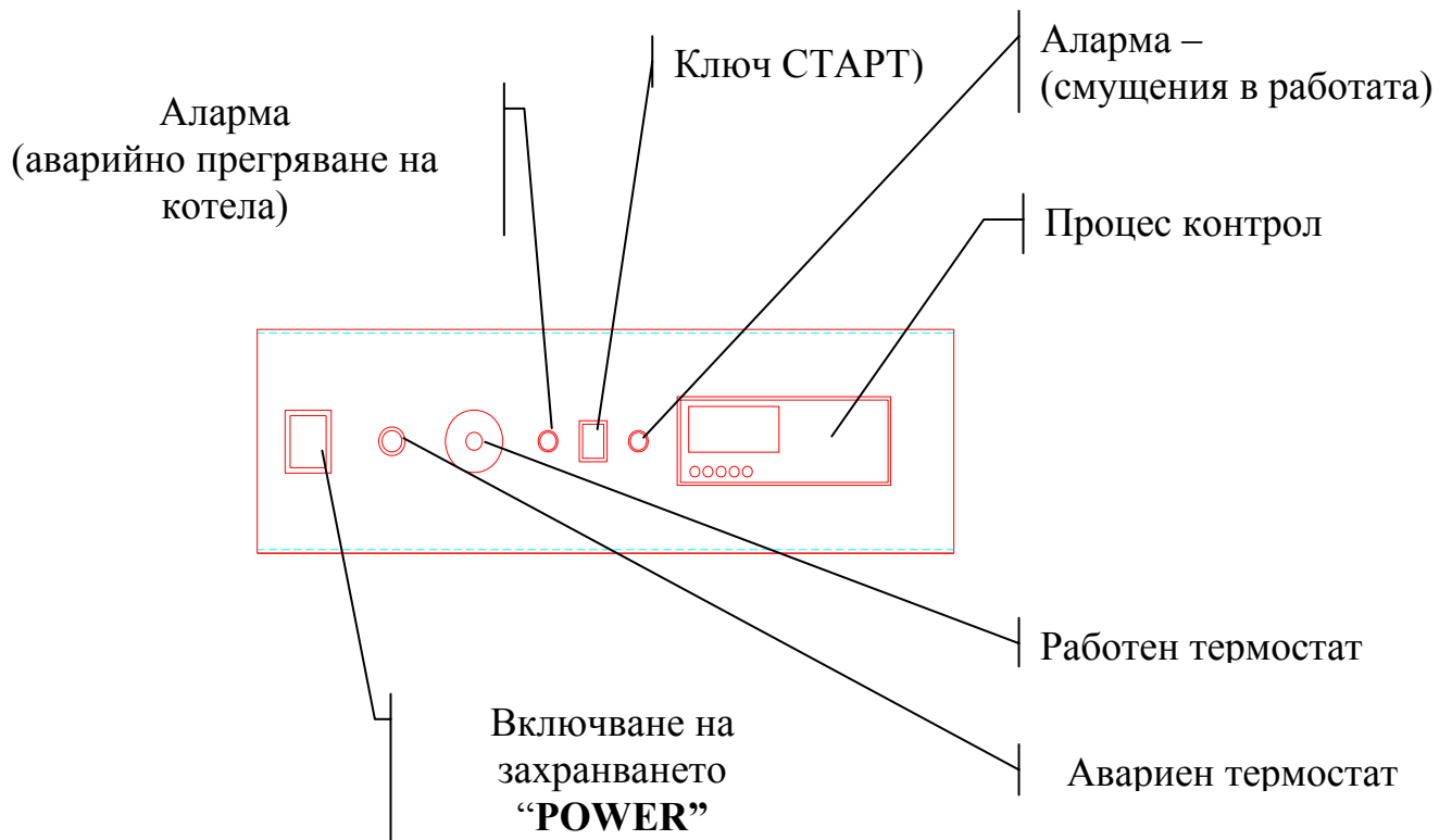
Фигура 1. Интерфейсно табло с контролни и управляващи уреди на водогреен пелетен котел “ЕРАТО Пелетерм 25 автоматичен”.
