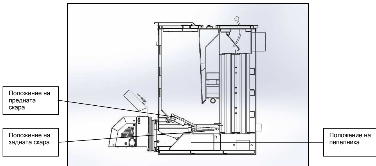
Фигура 12. Разположение на пепелника и скарите при работа на дърва при котли серия BiSolid Saver A
