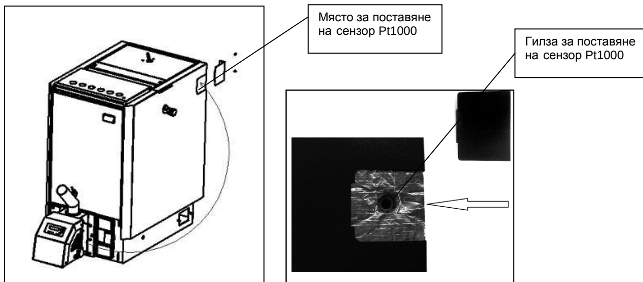
Фигура 16. Монтаж на сензора за температура на водата
