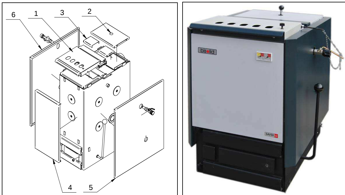
Фигура 17. Монтаж на капацие върху котелното тяло
