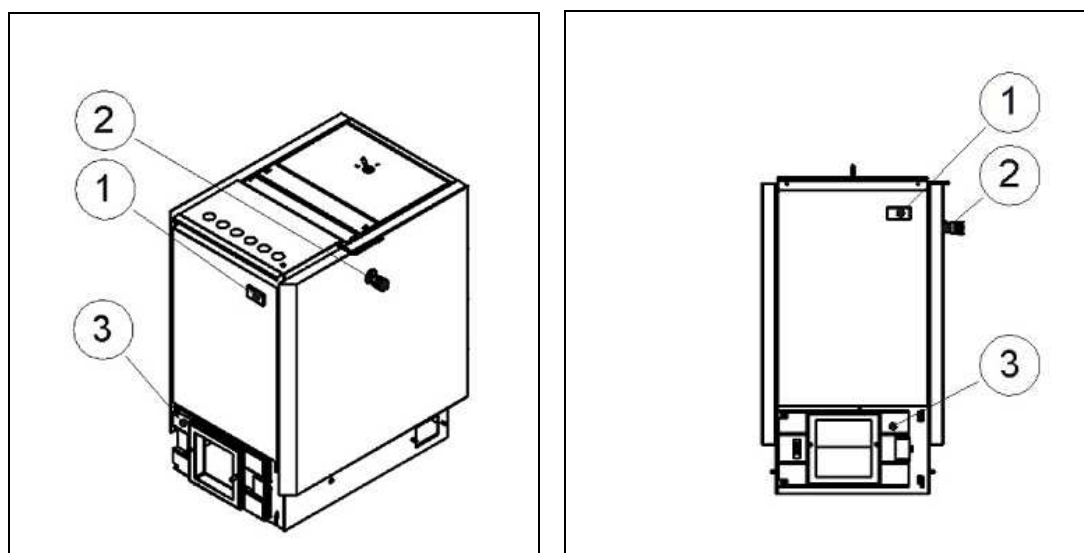
Фигура 8. Окомплектовка на котли от серия BiSolid Saver A
