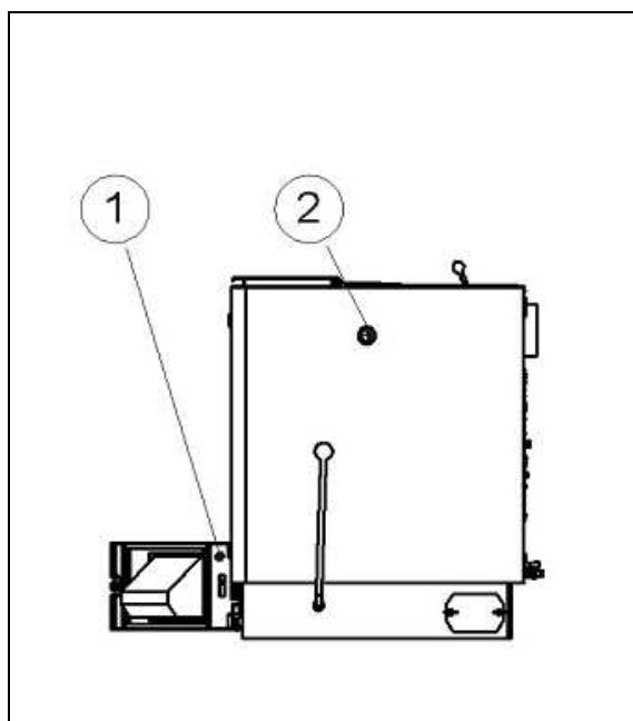
Фигура 6. Окомплектовка на котли от серия BiSolid Saver C
